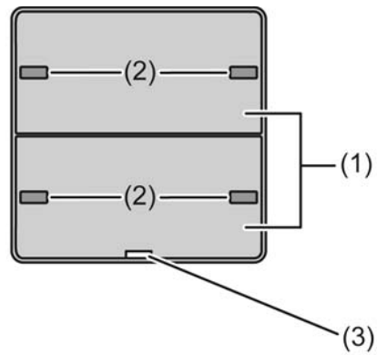
Bild 2: Geräteaufbau Tastsensor Komfort 2fach
